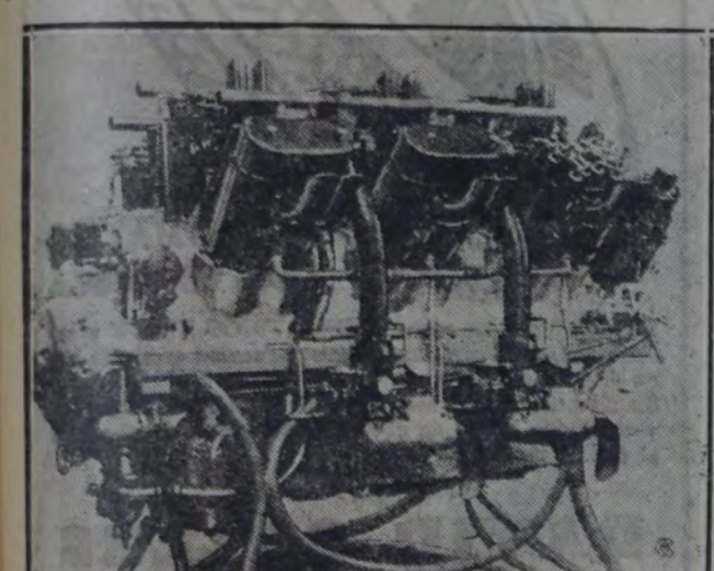
Motor Farman, 18 cilindros en W a 40°, 800 HP., a 1800 revoluciones por minuto
